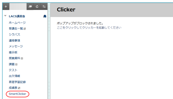
図 3 SmartClicker の起動
